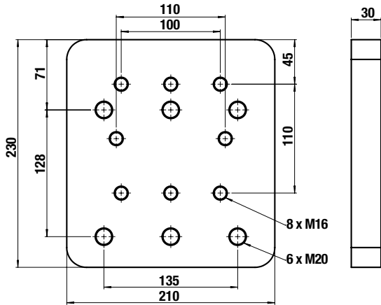
T520 0400 ÉPAISSEUR 30 POUR T2901100
