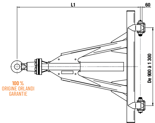
REPRÉSENTATION AVEC ANNEAUX BNA T4685035 EN OPTION
