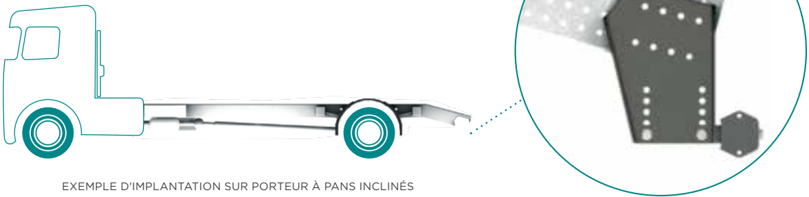
EXEMPLE D'IMPLANTATION SUR PORTEUR À PANS INCLINÉS
