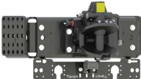
EXEMPLE DE MONTAGE SOUS TRAVERSE FIN DE CHÂSSIS MD, AVEC CROCHET BNA MANUEL, SUPPORT CAMÉRA ET CAMÉRA
