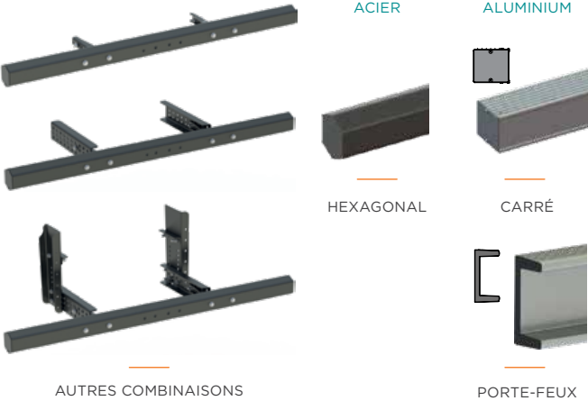
AUTRES COMBINAISONS POSSIBLES
