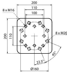
PS700 POUR OC68F8E & DIN50
