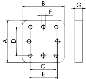
PS700 POUR OC68F8E & DIN50
