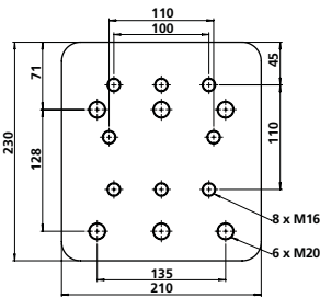
PS400 POUR GS911
