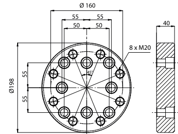
PS701 ADAPTEUR DIN50 / BNA
